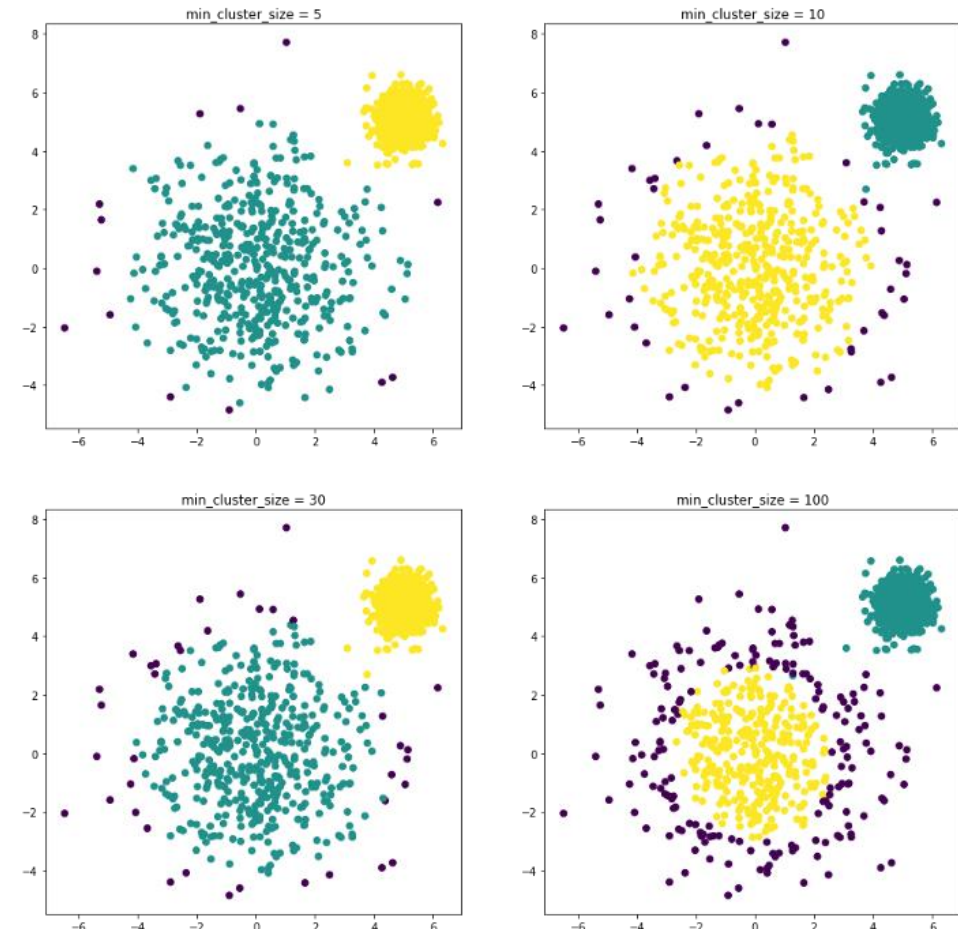
Hierarchical DBSCAN
